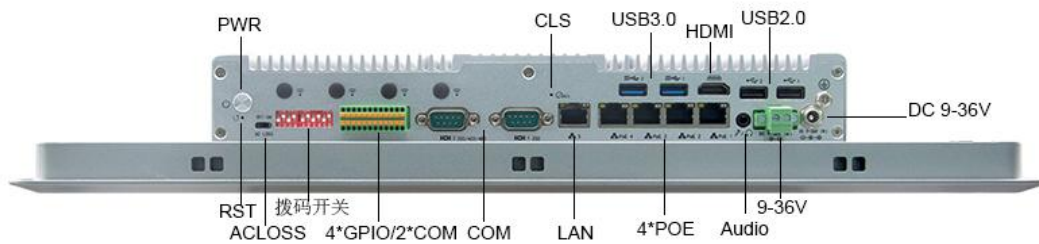
底部I/O视图
