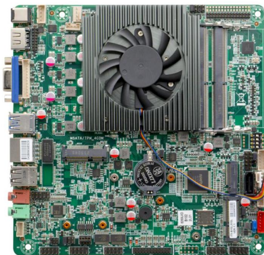
ITX-B101_I512L VER:1.1 主板正面图
